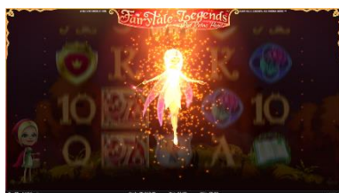
Funcțiile aleatorii
